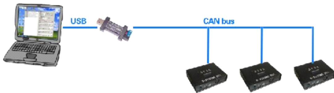
USB-CAN-B1转换器应用示意图
